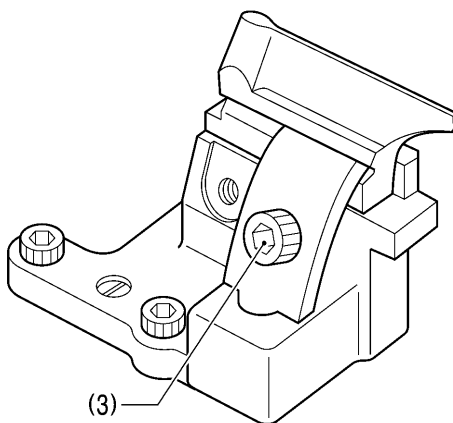
<-02-L1422、L1826、L2230 规格>
