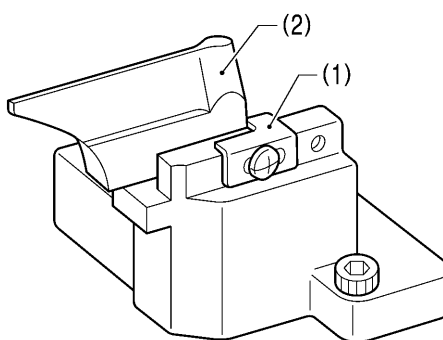
<-02-L1422、L1826、L2230 规格>
